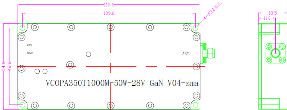
350-1000MHz Deawing
